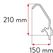
Faucet
